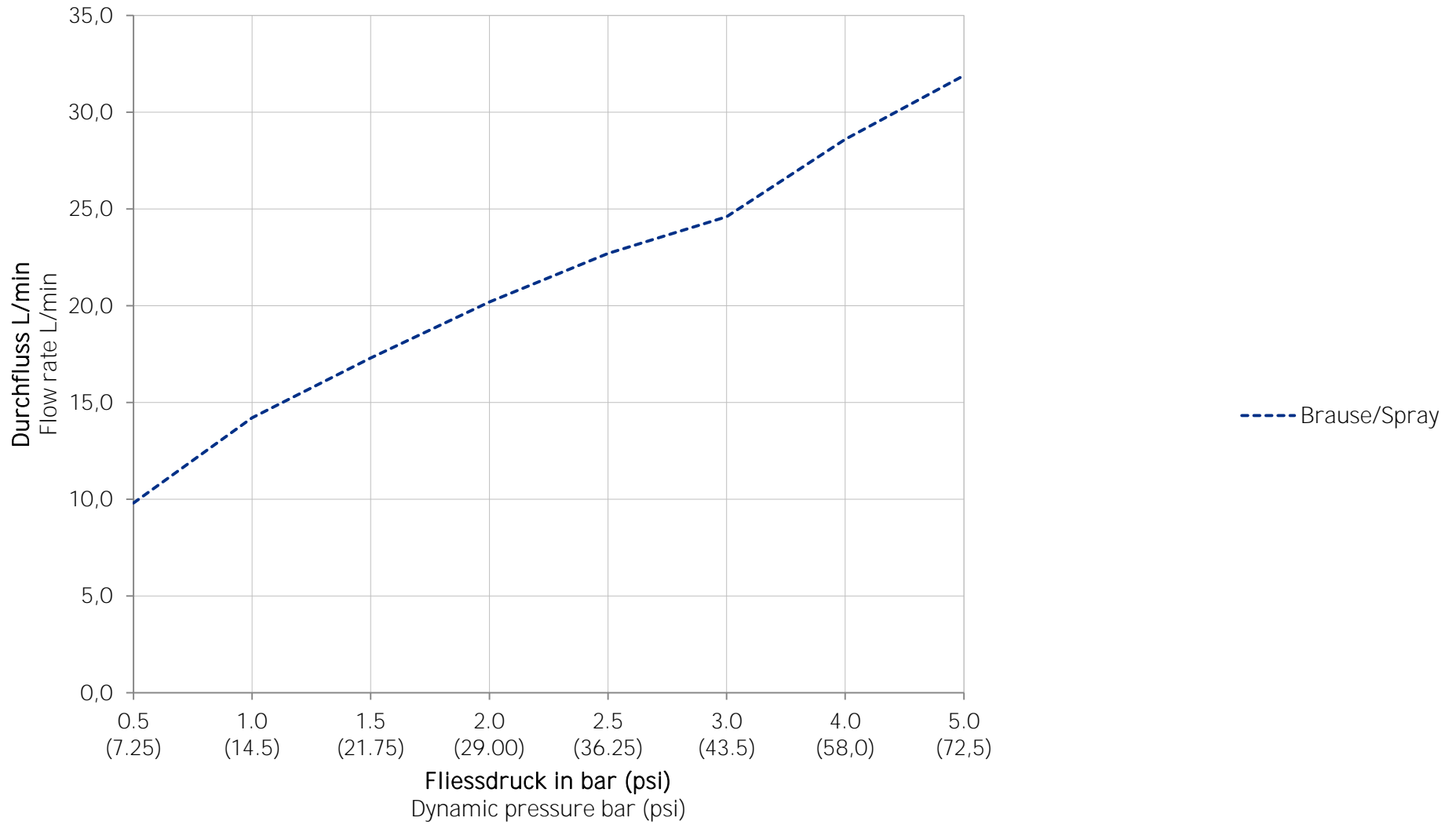
Durchflussdiagramm Mischwasser Flow rate chart mixed water
